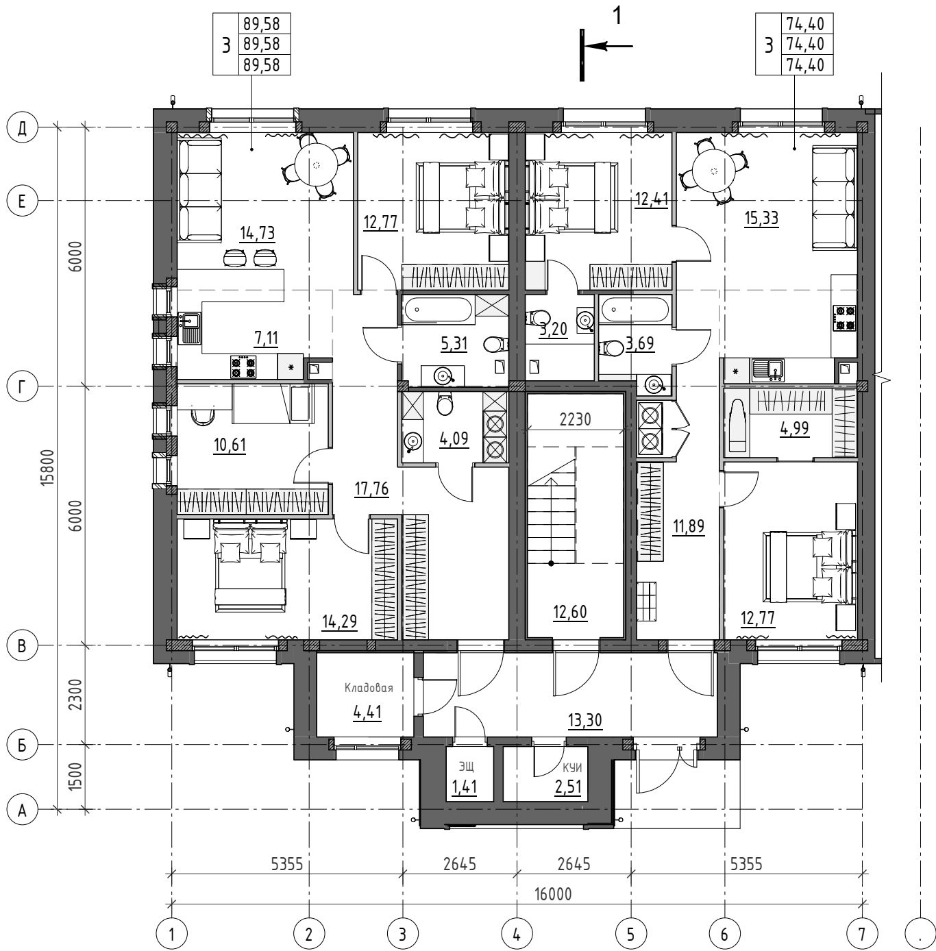
План этажа на отм. 0,000
