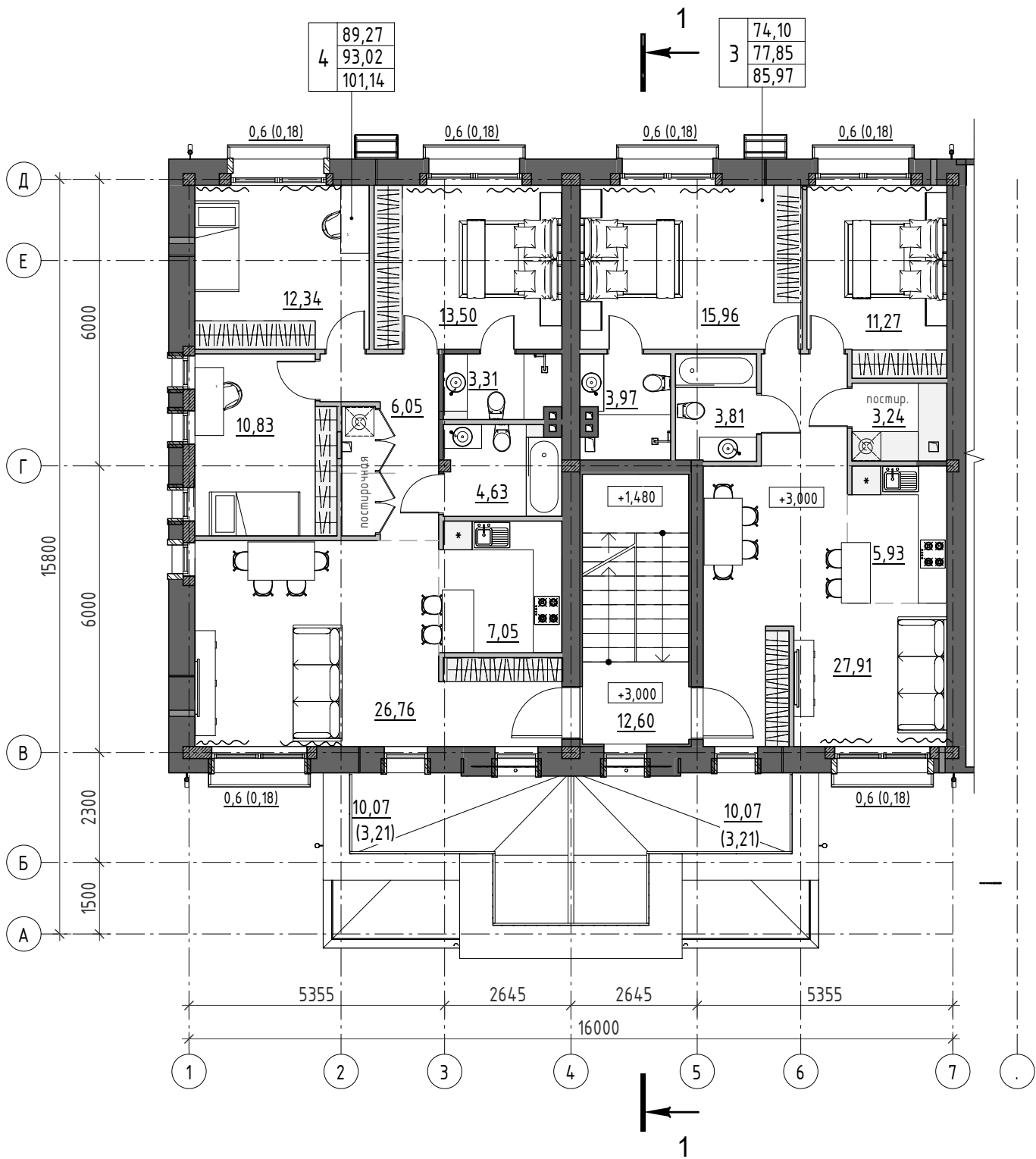
План этажа на отм. +3,000
