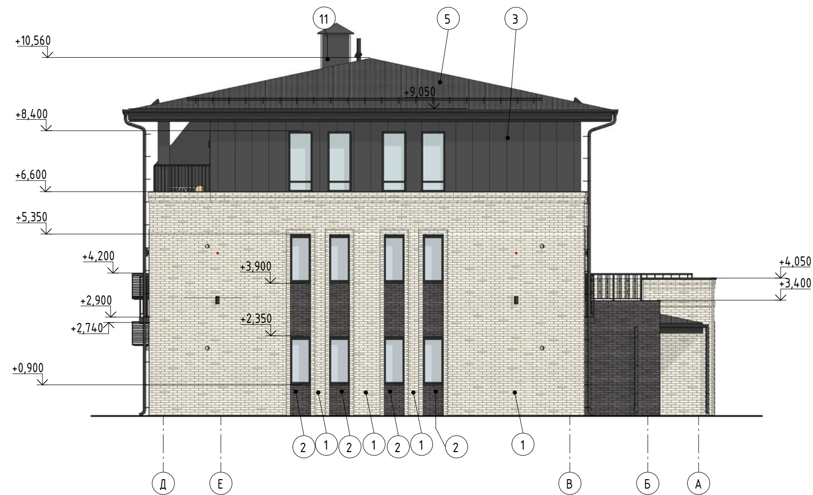
Фасад А-Д
